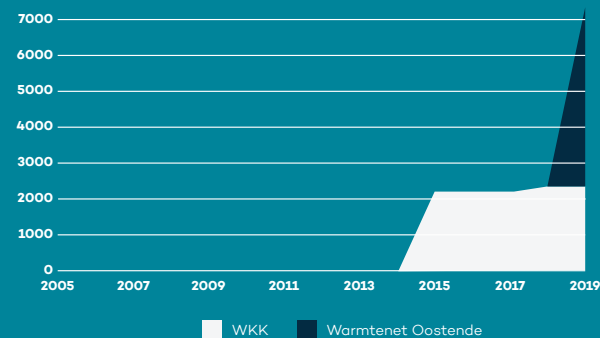
Evolutie thermisch vermogen in kW
