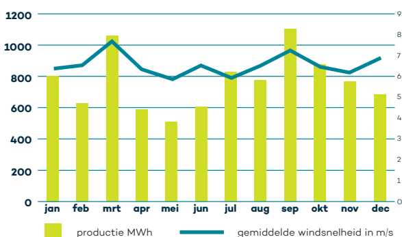
Wind: productie elektriciteit in MWh
