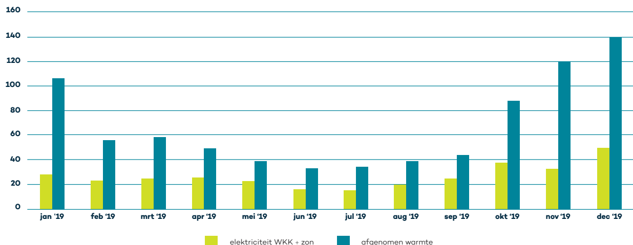
Stookplaats WZC Avondrust: elektriciteit (WKK + zon) en warmte in MWh
