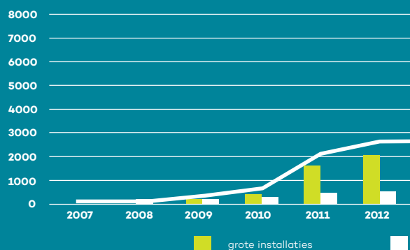
Aangroei zonne-installaties BeauVent in kWp
