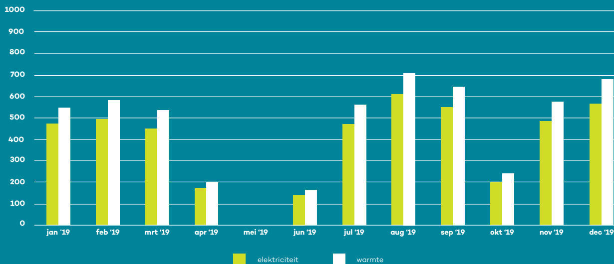
WKK Gramybel: elektriciteit en warmte in MWh
