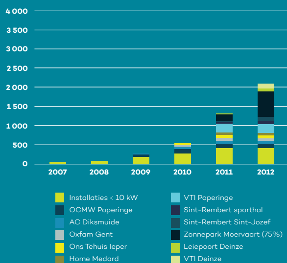
Overzicht productie per installatie in MWh
